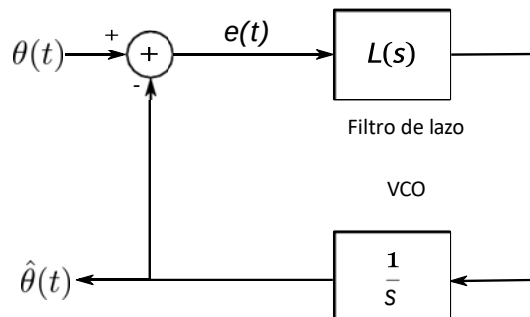
Figura 11: Diagrama en bloques de un PLL lineal.
