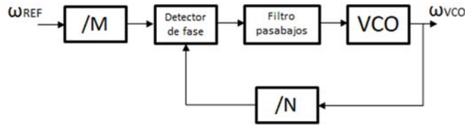
Figura 12: Sintetizador de frecuencia del Ejercicio 50.
