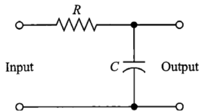
Figura 8: Filtro RC correspondiente al Ejercicio 33.
