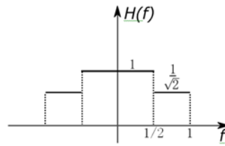
Figura 10: Respuesta en frecuencia del canal del Ejercicio 39.
