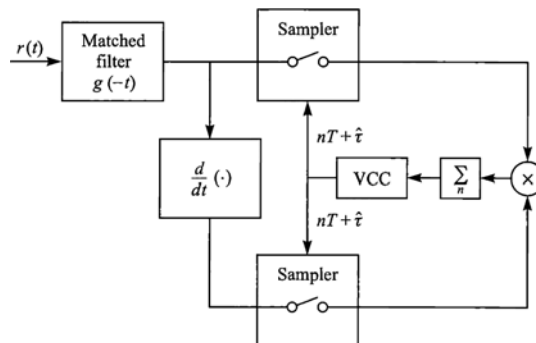
Figura 13: Implementación alternativa del sincronizador Early-Late .
