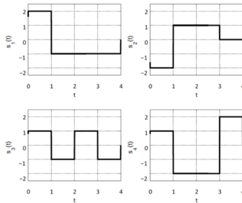
Figura 1: Señales correspondientes al Ejercicio 3.
